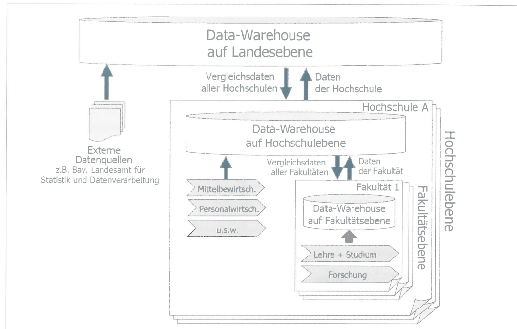
Abb. 3: Architektur des Data-Warehouse-Systems von CEUS
